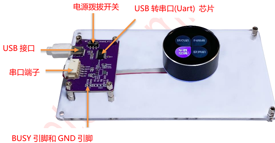
图 1-2：模块主要组件与接口
