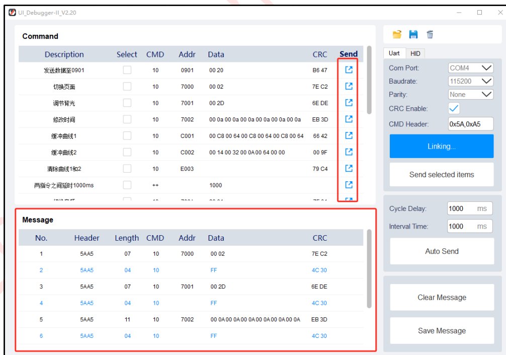
图 2-15：通过电脑与演示模块通讯
