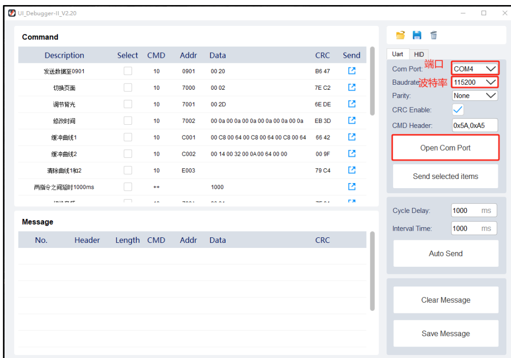
图 2-14：点击 Open Com Port 打开端口
