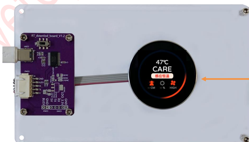
图 2-5: LT168A 应用-四合一功能（吹风机）演示画面 4
