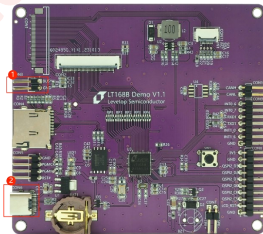
图 16.33：168B 接线示意
