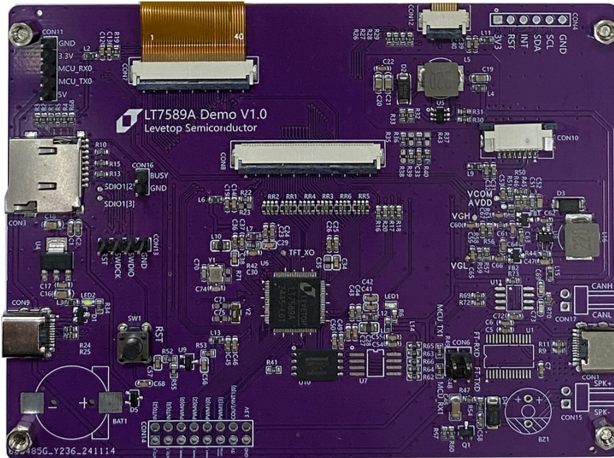
图 16-17: LT7589B 串口屏的开发演示板 (Demo Kit)
