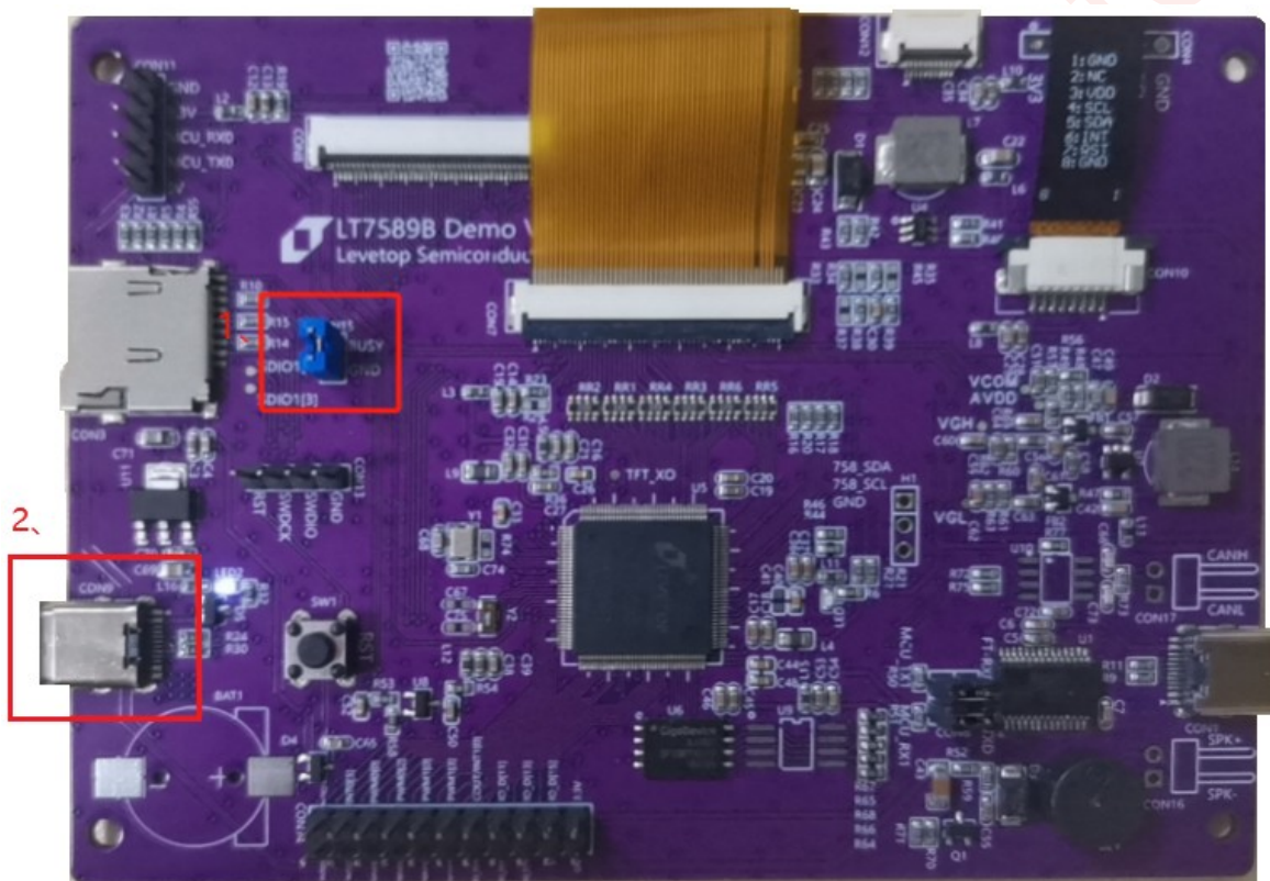
图 16-11：LT7589 演示板及其接线说明
