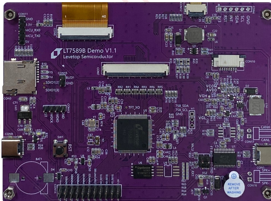
图 16-18: LT7589B 串口屏的开发演示板 (Demo Kit)
