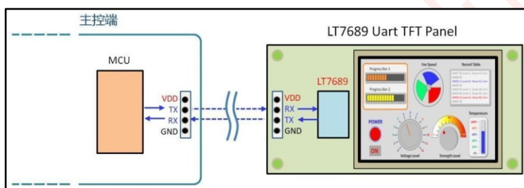
图 1-1：主控端 MCU 的 Uart 串口对 TFT 串口屏进行通信
