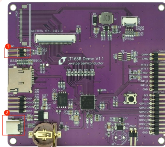
图 16-55：168B 接线示意
