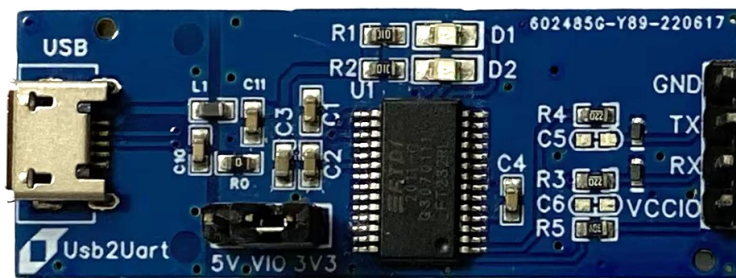
图 16-24: USB 转 TTL 模块
