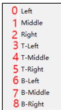
图 10-49: 对齐方式
