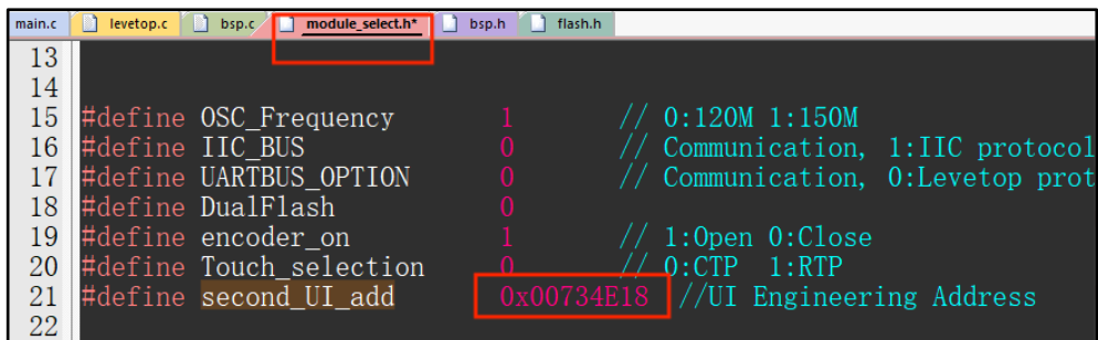
图 13-13: 填入 second_UI_add
