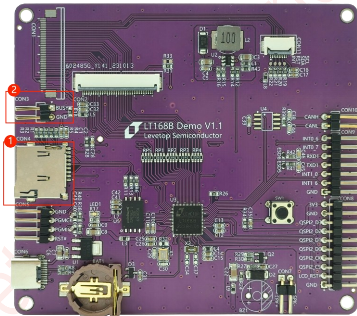
图 16-37: LT168B 示意图
