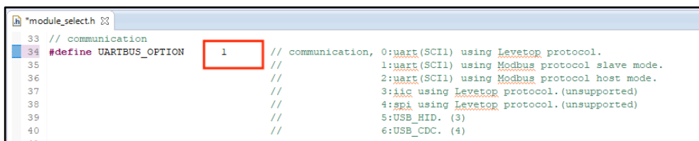
图 11-6：LT168 选择 modbus 从机模式
