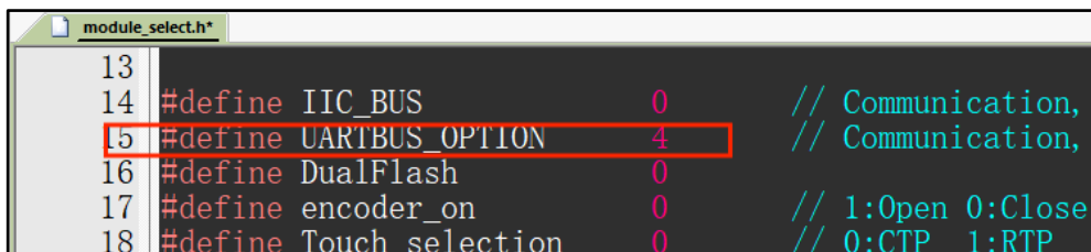
图 12-6: 选择 Vcom 通信模式
