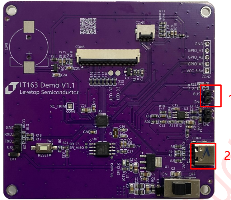
图 2-9: LT163 接线示意图
