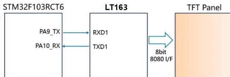
图 3-2：主控端 MCU (STM32F103RCT6) 用串口与 LT163 串口屏芯片通讯
