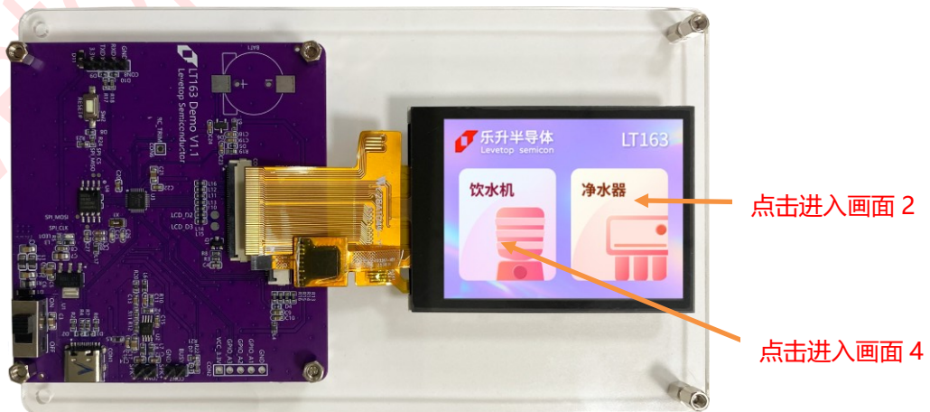
图 2-2：LT163 应用-饮水机 / 净水器演示画面 1
