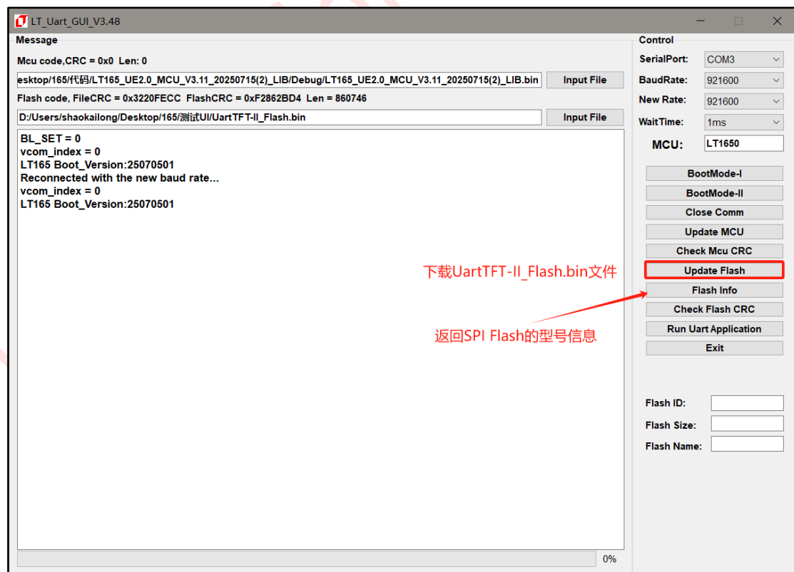
图 2-12: 烧录 UartTFT-II_Flash.bin
