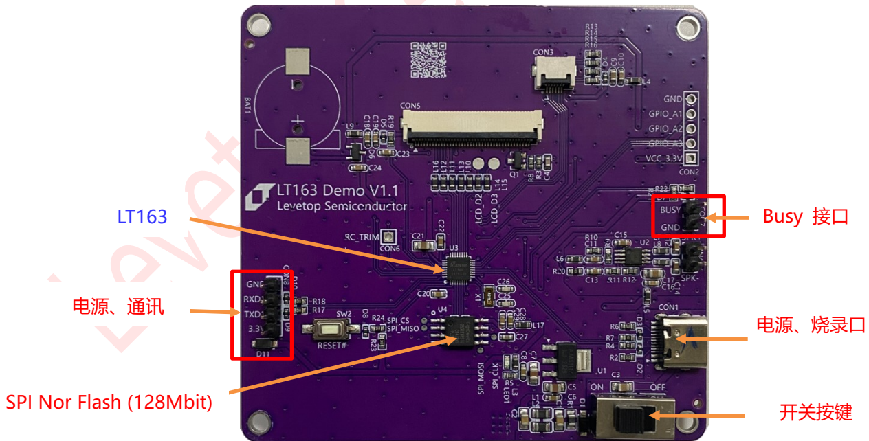
图 1-2: 模块主要组件与接口
