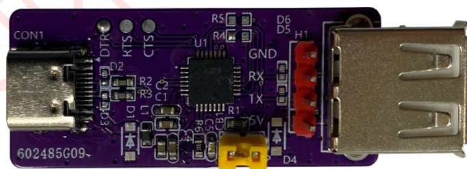
图 4-2: LT_Uart_ISP 小板
