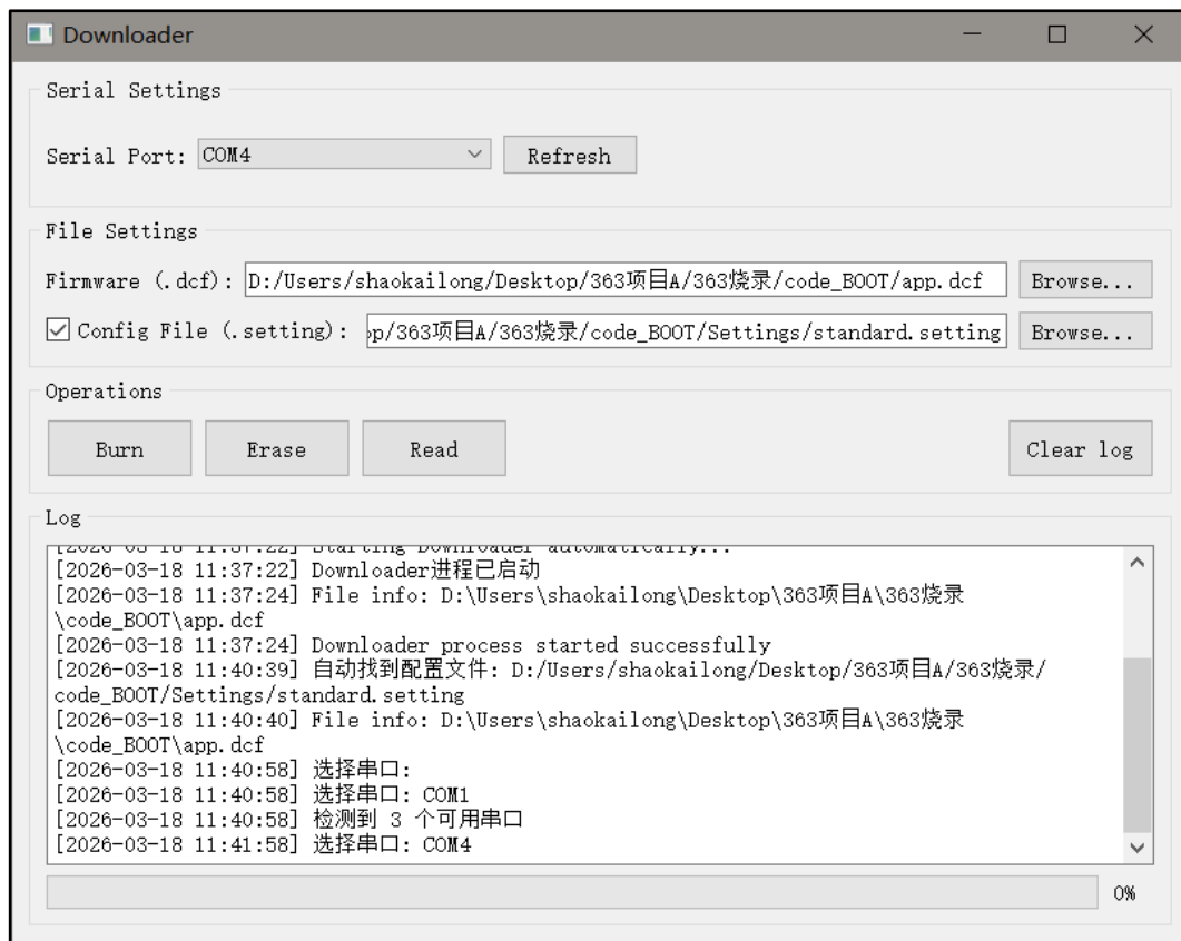
图 4-3：连接烧录端口
