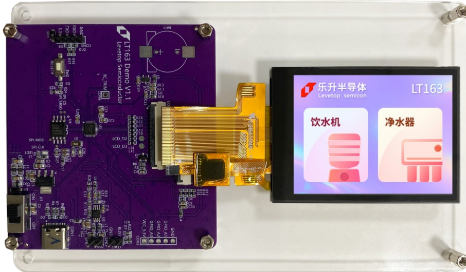
图 1-1: 演示模块外观图
