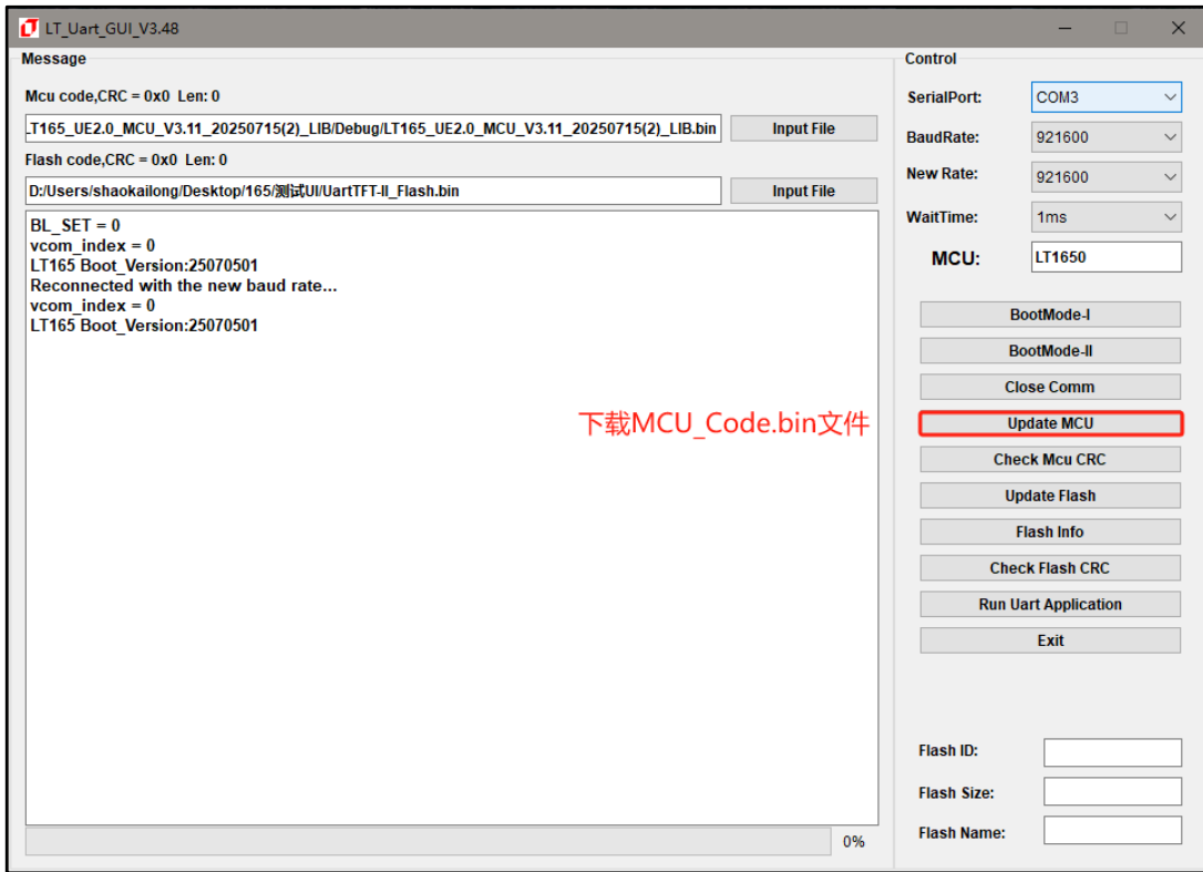
图 2-24: 烧录 MCU_Code.bin
