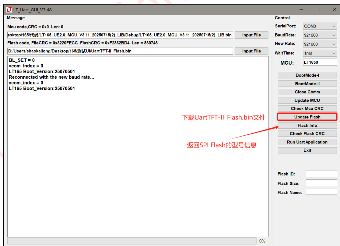
图 2-11：烧录 UartTFT-II_Flash.bin
