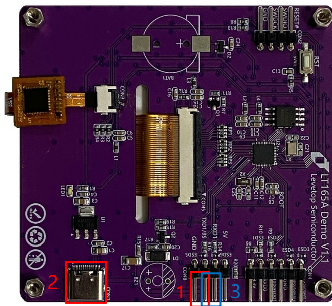
图 2-8: LT165A 接线示意图
