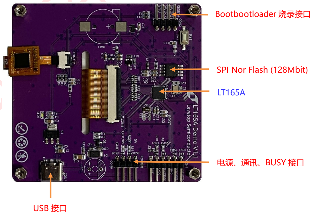
图 1-2: 模块主要组件与接口
