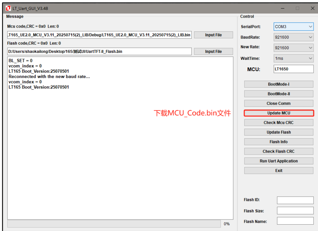
图 2-23：烧录 MCU_Code.bin
