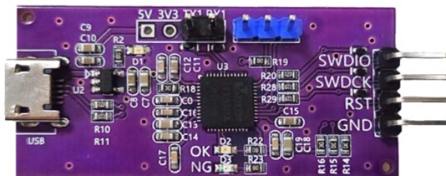
图 4-2: LT_SWD_ISP_Programmer_Lite 烧录器
