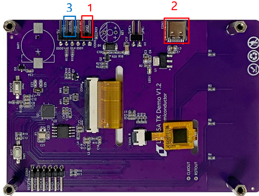
图 2-8: LT165A 接线示意图
