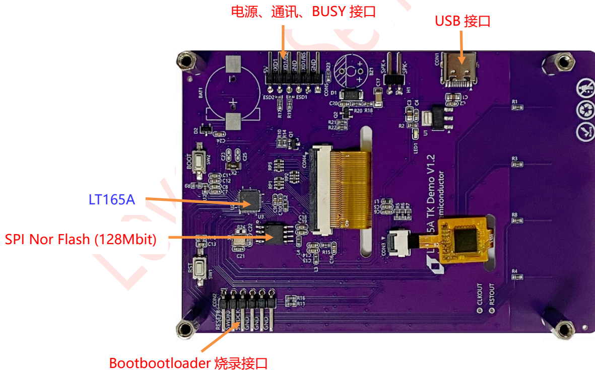
图 1-2: 模块主要组件与接口
