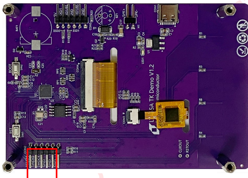
图 4-1: LT165A 演示模块
