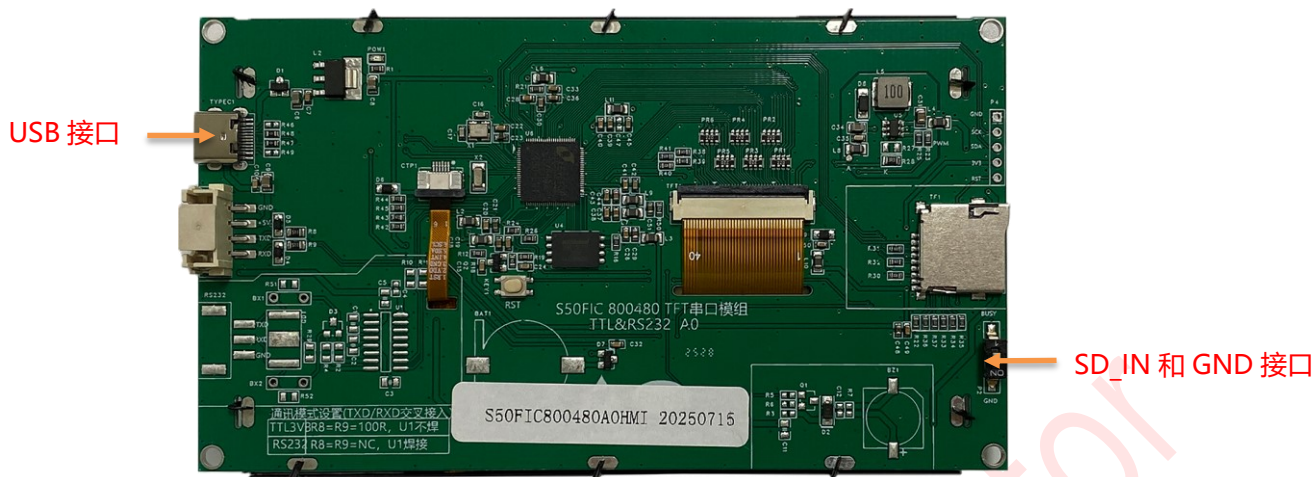
图 2-13: LT7589 演示板及其接线说明
