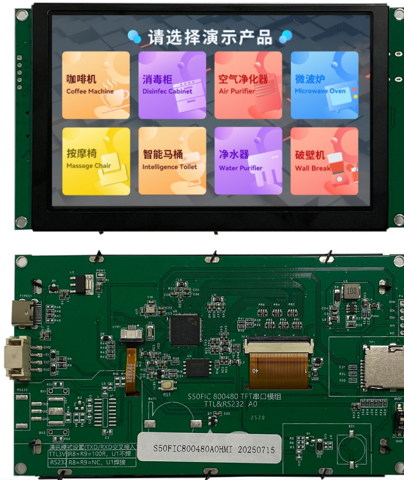
图 1-1: LT7589A (M7589A-50-0800480-SCX-GZ-VA0) 演示模块外观图
