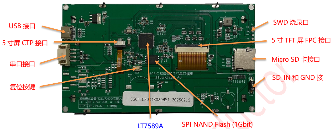
图 1-2: LT7589A 控制板主要组件与接口
