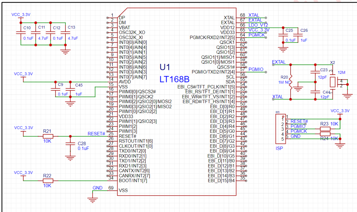
图 7-1: LT168B 的外围相关电路
