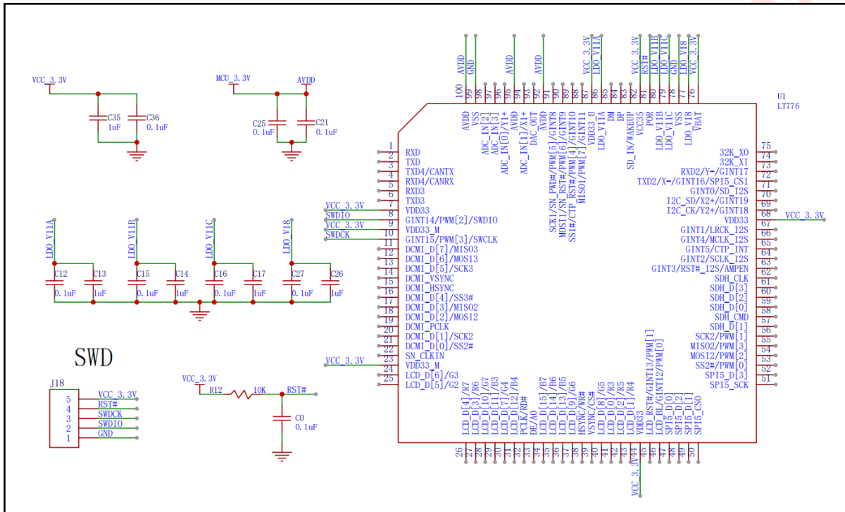
图 9-1: LT776 的外围相关电路
