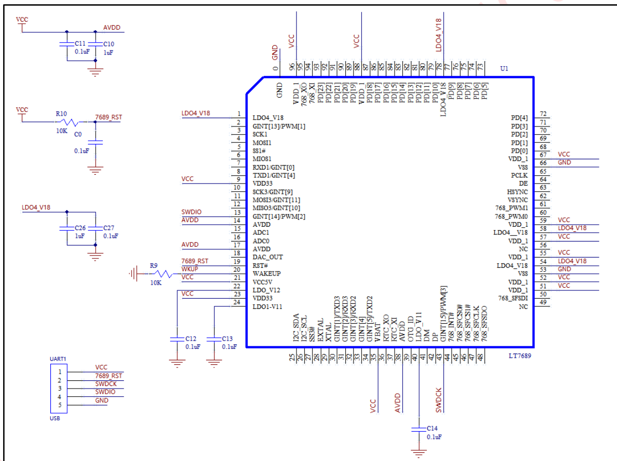
图 8-1: LT7689 的外围相关电路
