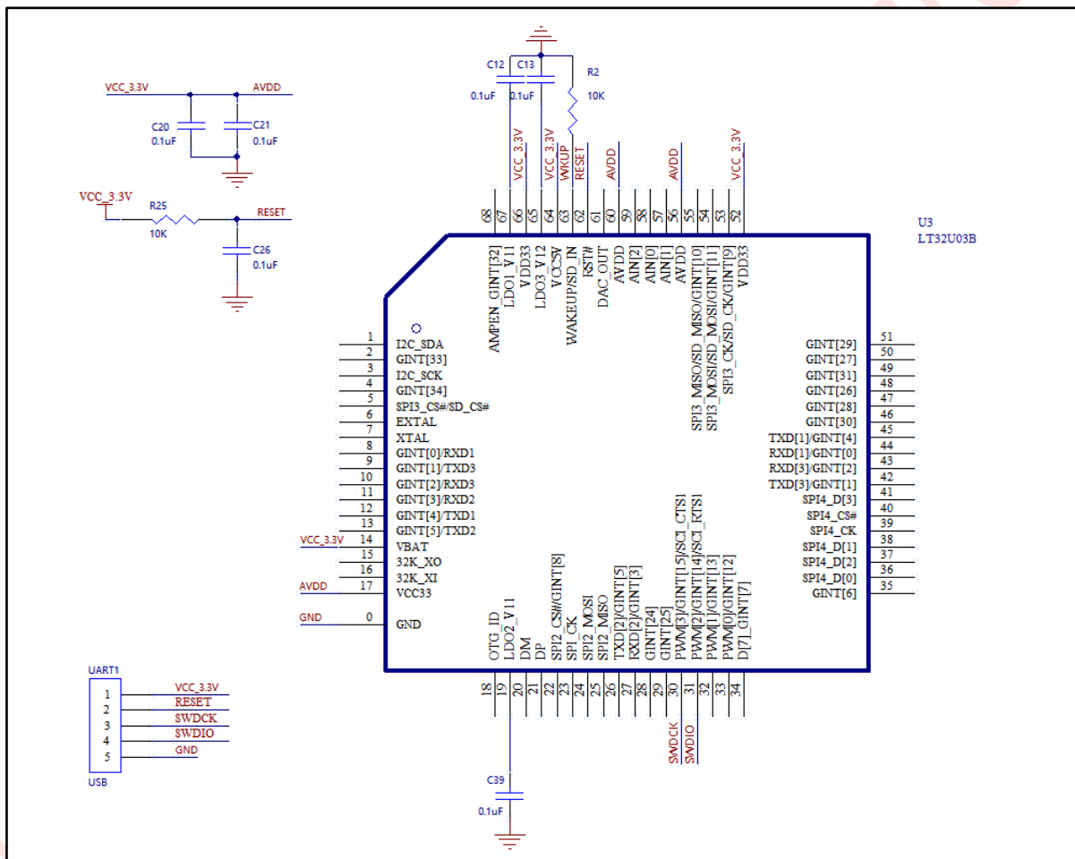
图 11-1: LT32U03B 的外围相关电路
