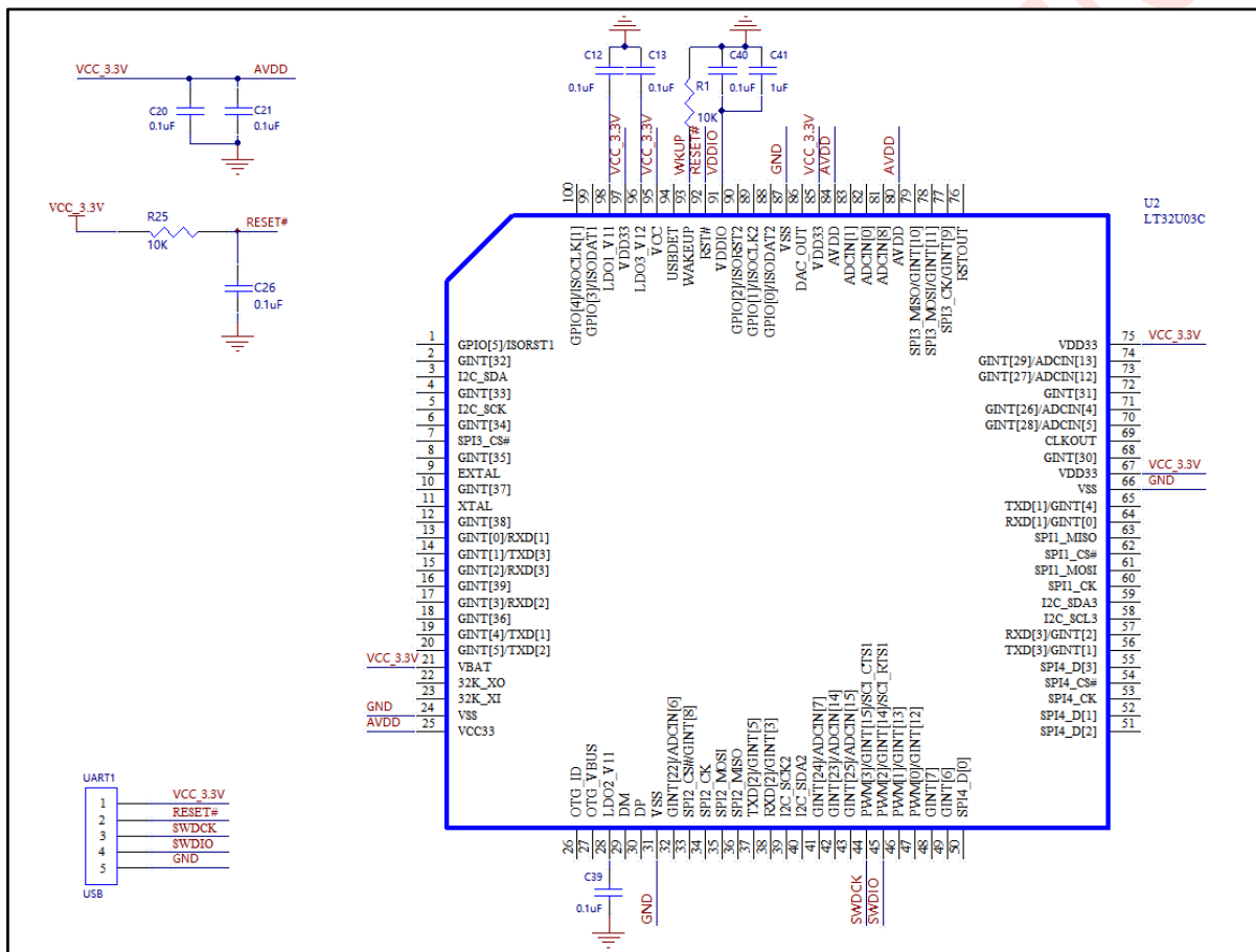
图 12-1: LT32U03C 的外围相关电路
