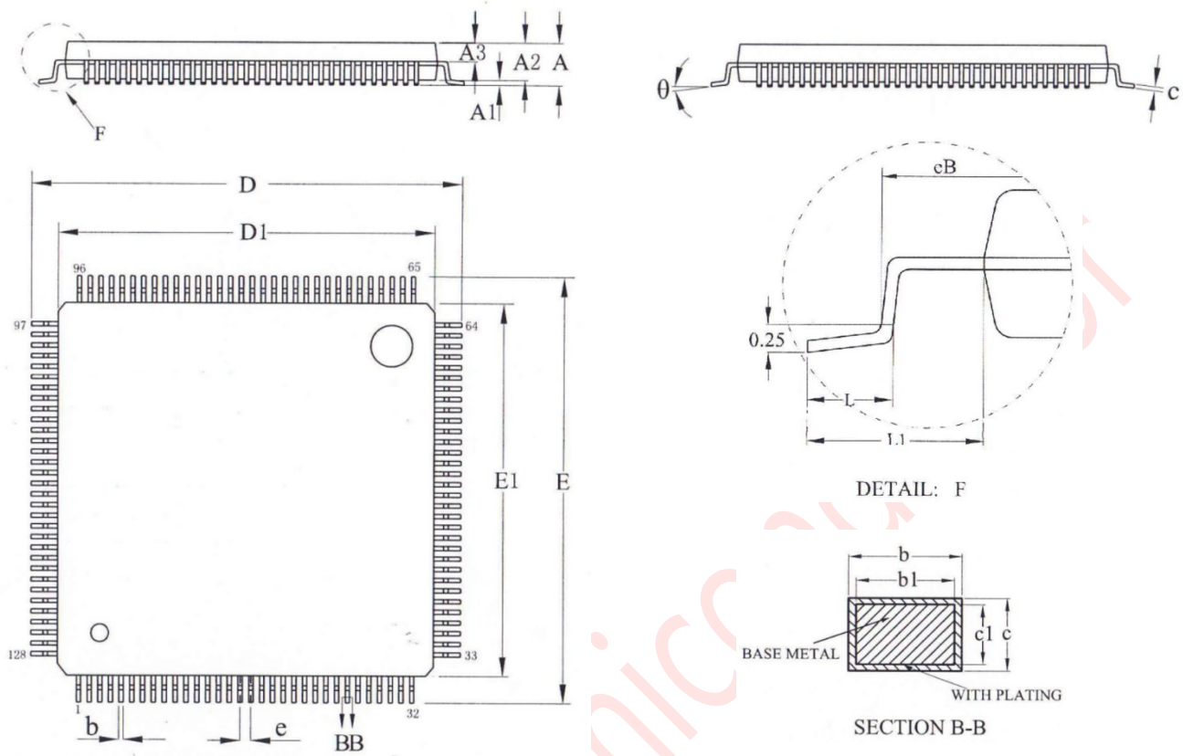
图 8-2: LQFP-128Pin 外观尺寸图
