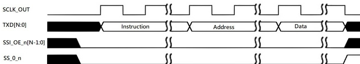
图 21-37: 典型的写入操作双/四/八进制 SPI 模式
