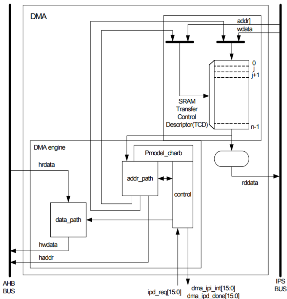
图 13-1: DMA 结构图
