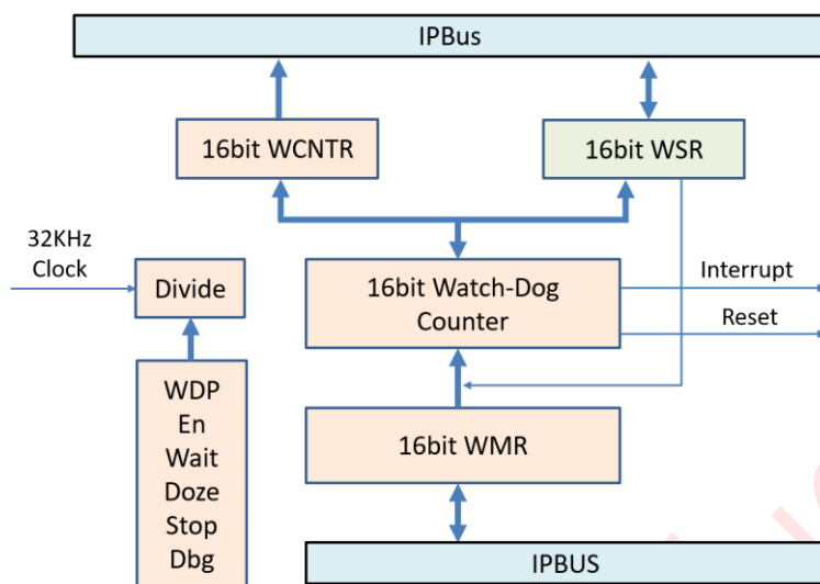
图 16-1: 看门狗定时器方块图
