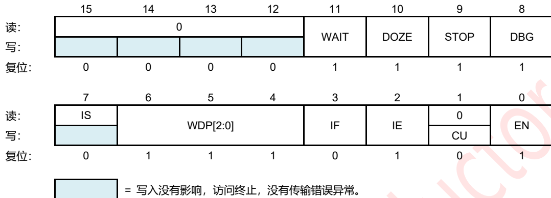
图 16-3: 看门狗控制寄存器 (WCR)
