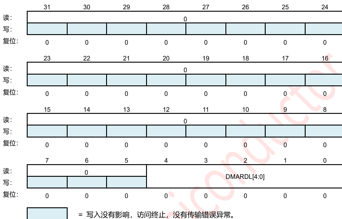
图 21-23: DMA 接收数据级别 (DMARDLR)
