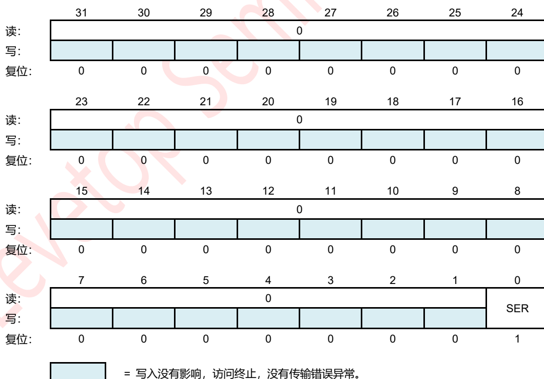
图 21-33: XIP 从属服务器启用寄存器 (XIPSER)
