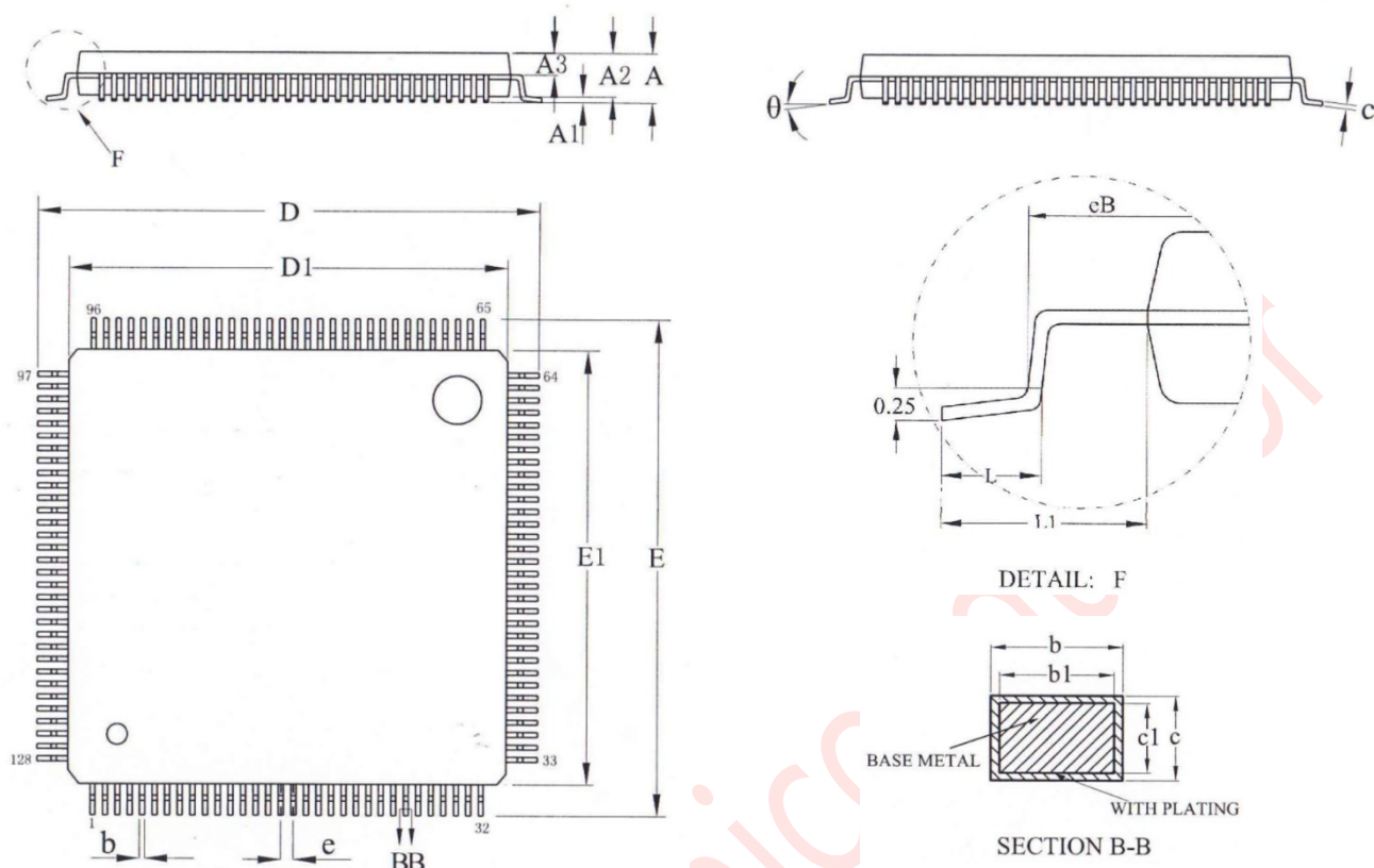
图 28-2: LQFP-128Pin 外观尺寸图
