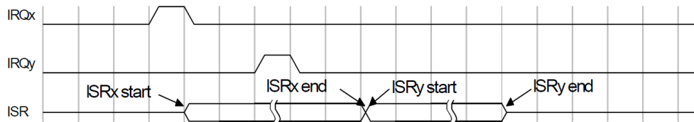
图 7-10：具有冲突的较低优先级中断
