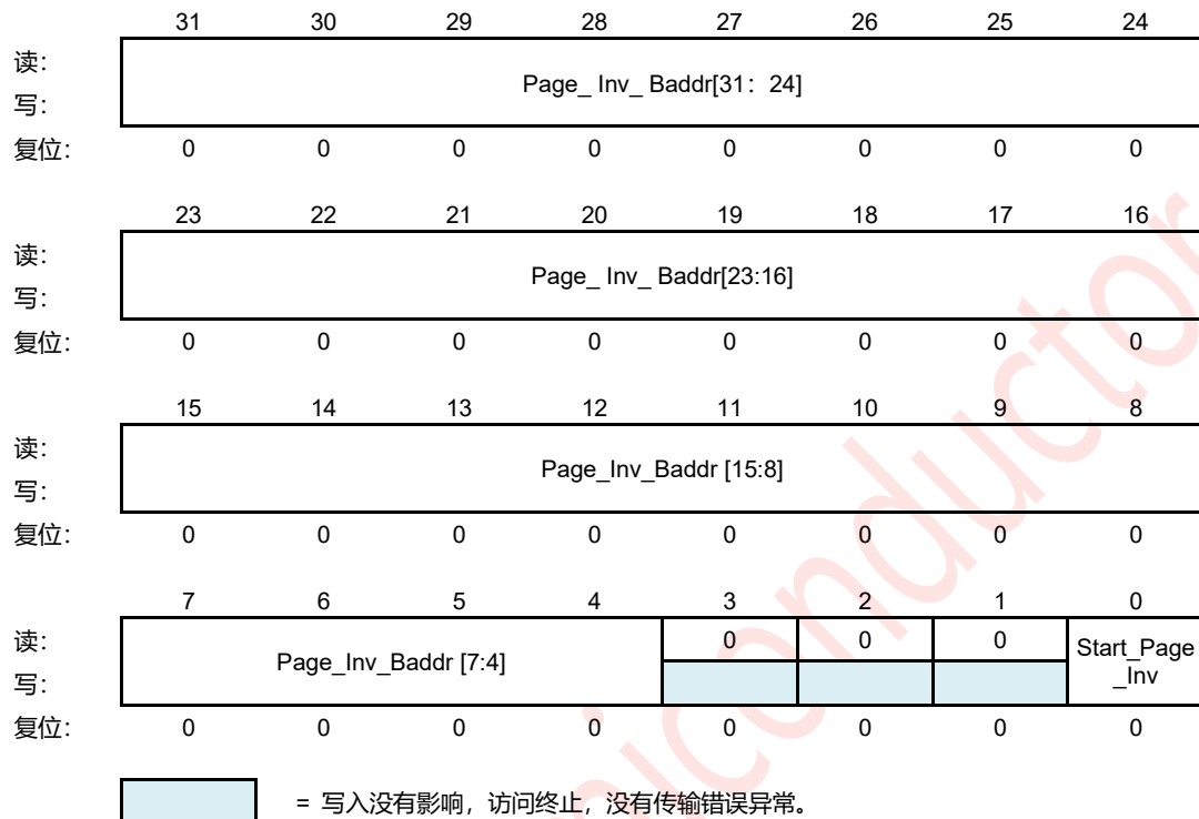
图 12-7: 高速缓存页不验证基本地址寄存器 (LMEM_PAGE_INV_BADDR)
