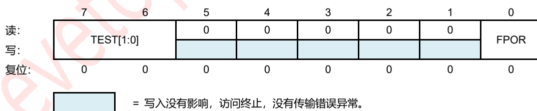
图 10-2: 复位测试寄存器（RTR）
