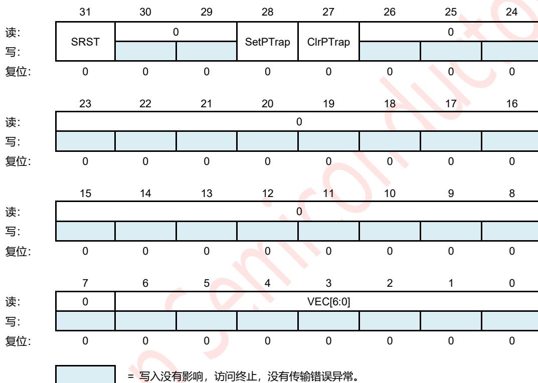
图 7-1: 中断控制状态寄存器 (ICSR)
