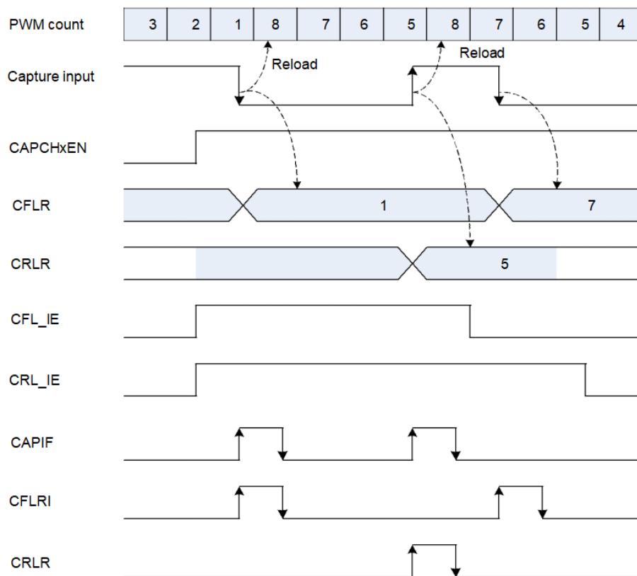
图 22-26: 捕获基本计时器操作
