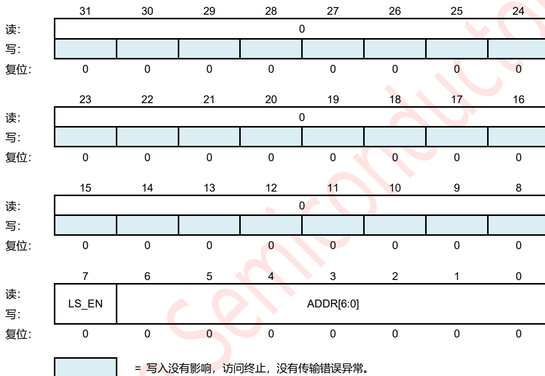
图 24-9: 地址寄存器 (ADDR)
