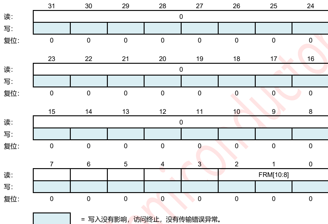
图 24-12: 帧数寄存器 (FRMNUMH)
