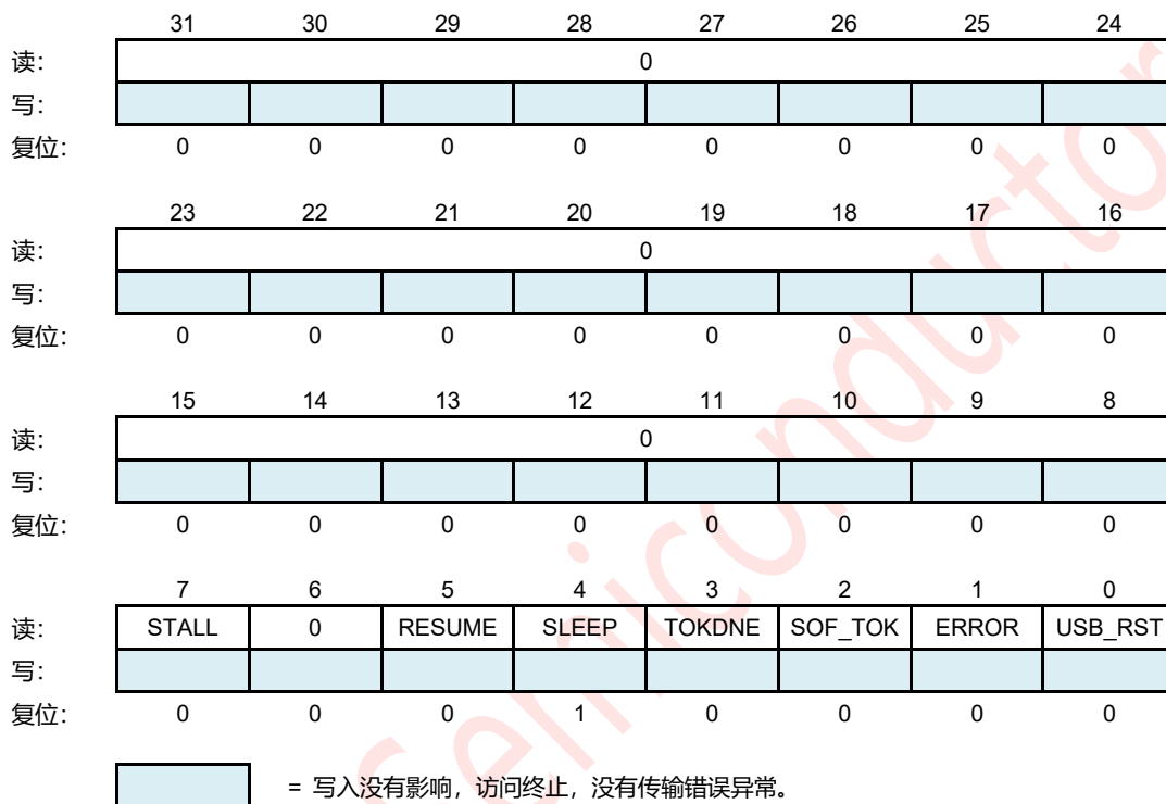
图 24-3: 中断状态寄存器 (INT_STAT)
