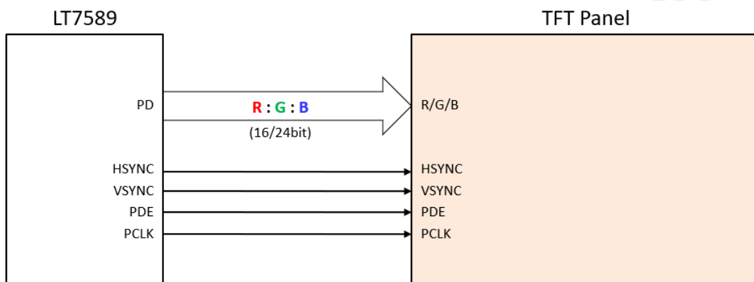
图 3-5: LT7589 与 TFT LCD 屏的连接
