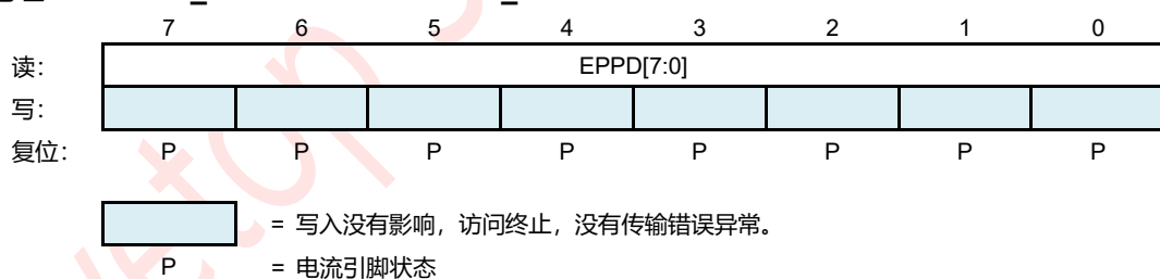
图 18-7: EPOR 端口引脚数据寄存器 (EPPDR)
